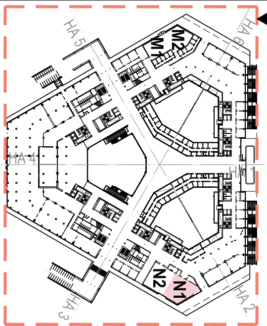
VERORTUNG SAAL N1 M 1/2000
